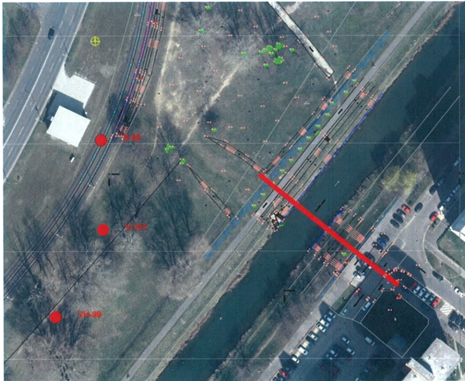
Lávka č.2 Situácia dokumentačných bodov základného prieskumu s archívnymi sondami v mieste projekčného zámeru
